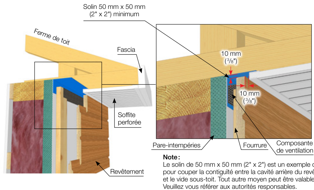
a) Avec débord de toit
