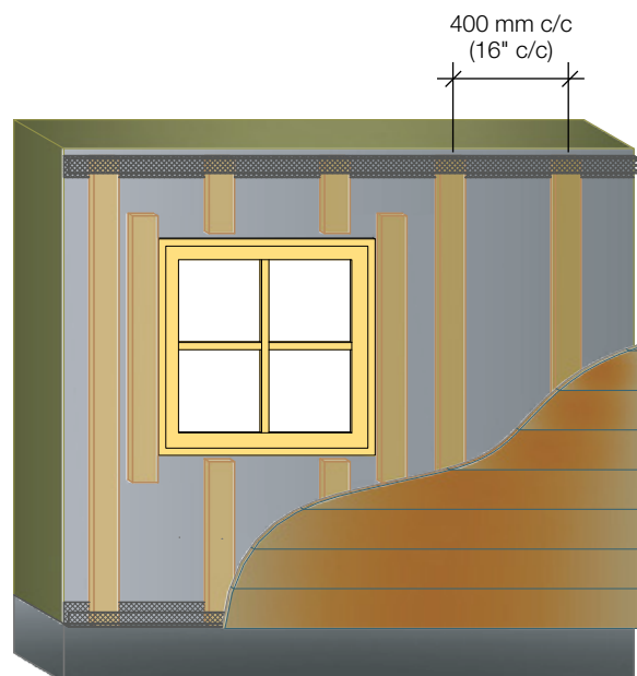
FIGURE 4 • Disposition des fourrures pour le revêtement horizontal
