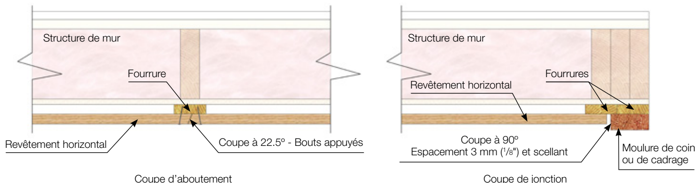
FIGURE 18 • Coupe à effectuer aux joints d'aboutement et de jonction
