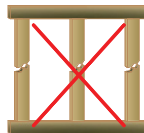
Fourrure horizontale au haut et au bas du mur à proscrire
